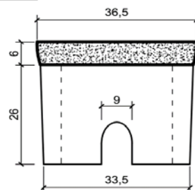
PERFIL
