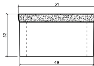
ELEVACIÓN
