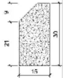
PERFIL
