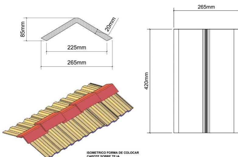
ISOMETRICO FORMA DE COLOCAR CAPOTE SOBRE TEJA.
