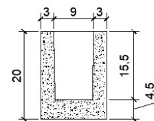
PERFIL
