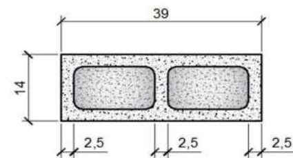
PLANTA
