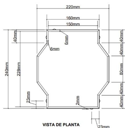
VISTA DE PLANTA
